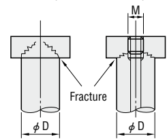
[Fig. 5] Flange fracture
