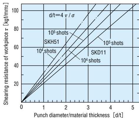
[Fig. 3] Punching limit
